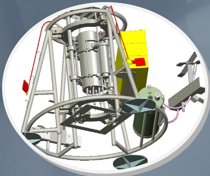
Aspirateur pour le prélèvement et détail de la pompe
