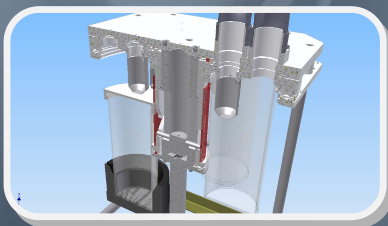
Aspirateur pour le prélèvement et détail de la pompe
